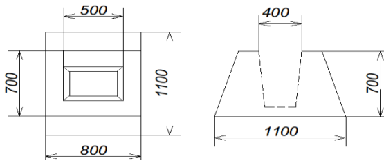
Фундамент Ф0
