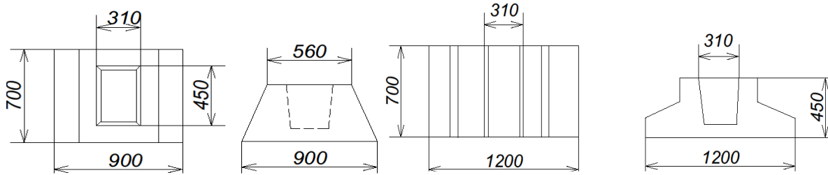
Фундамент Ф0
